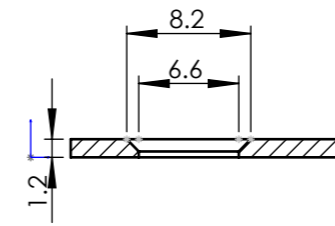
SECTION I-I SCALE 2 : 1
